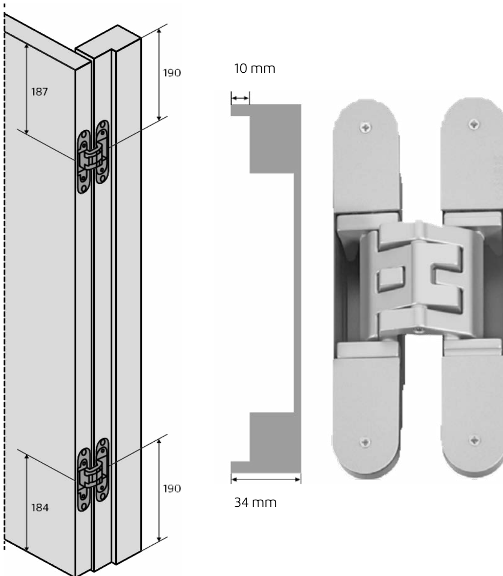
Kubica (blinde) scharnieren. Vaste maten scharnierkrozing
